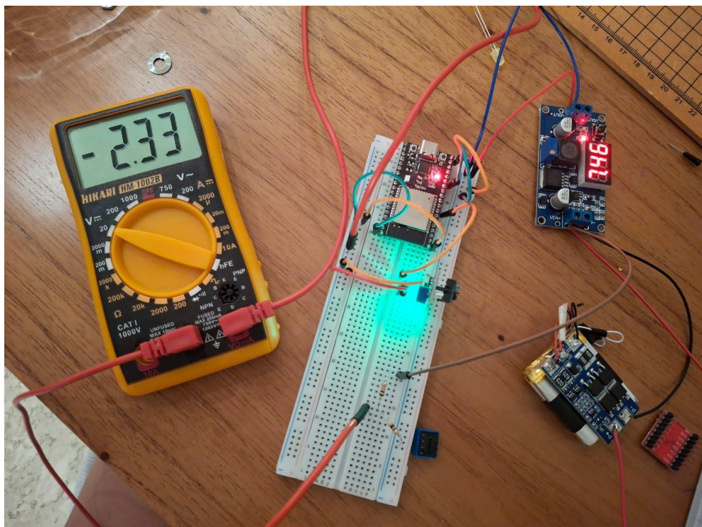
Figura 2 – Leitura da saída do Divisor de Tensão
